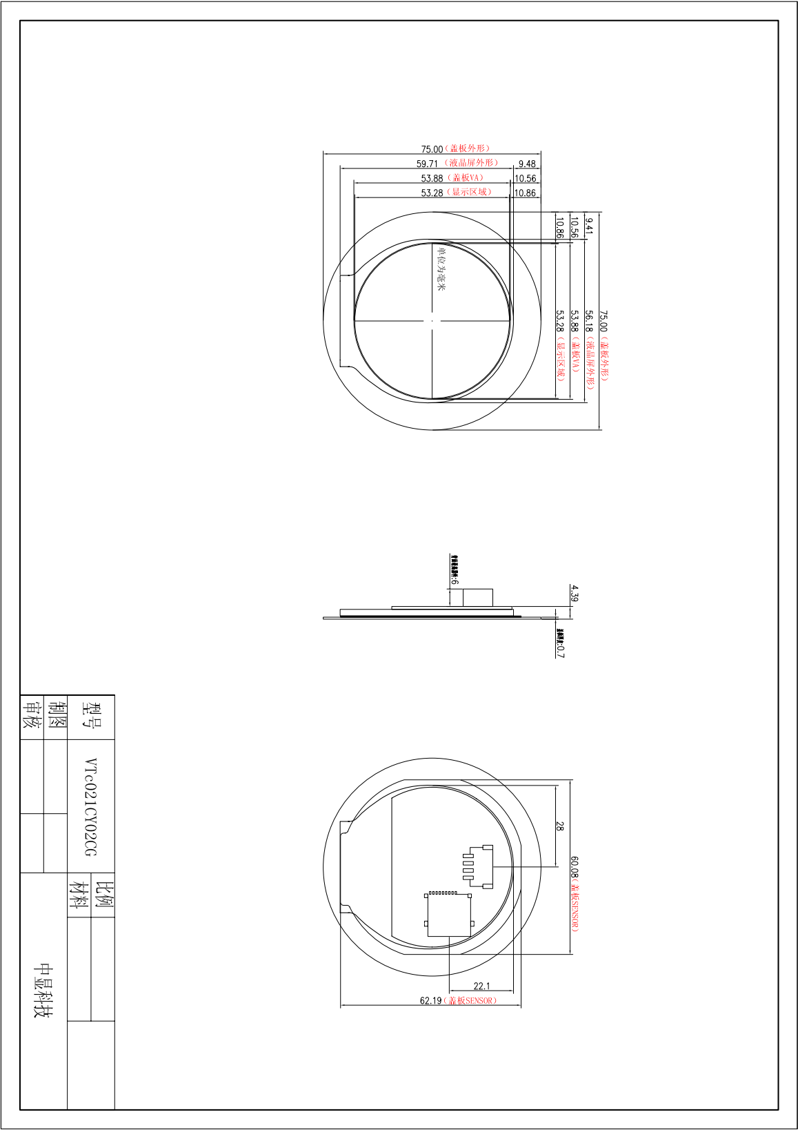
图 2 VTc021CY02CG 尺寸图
